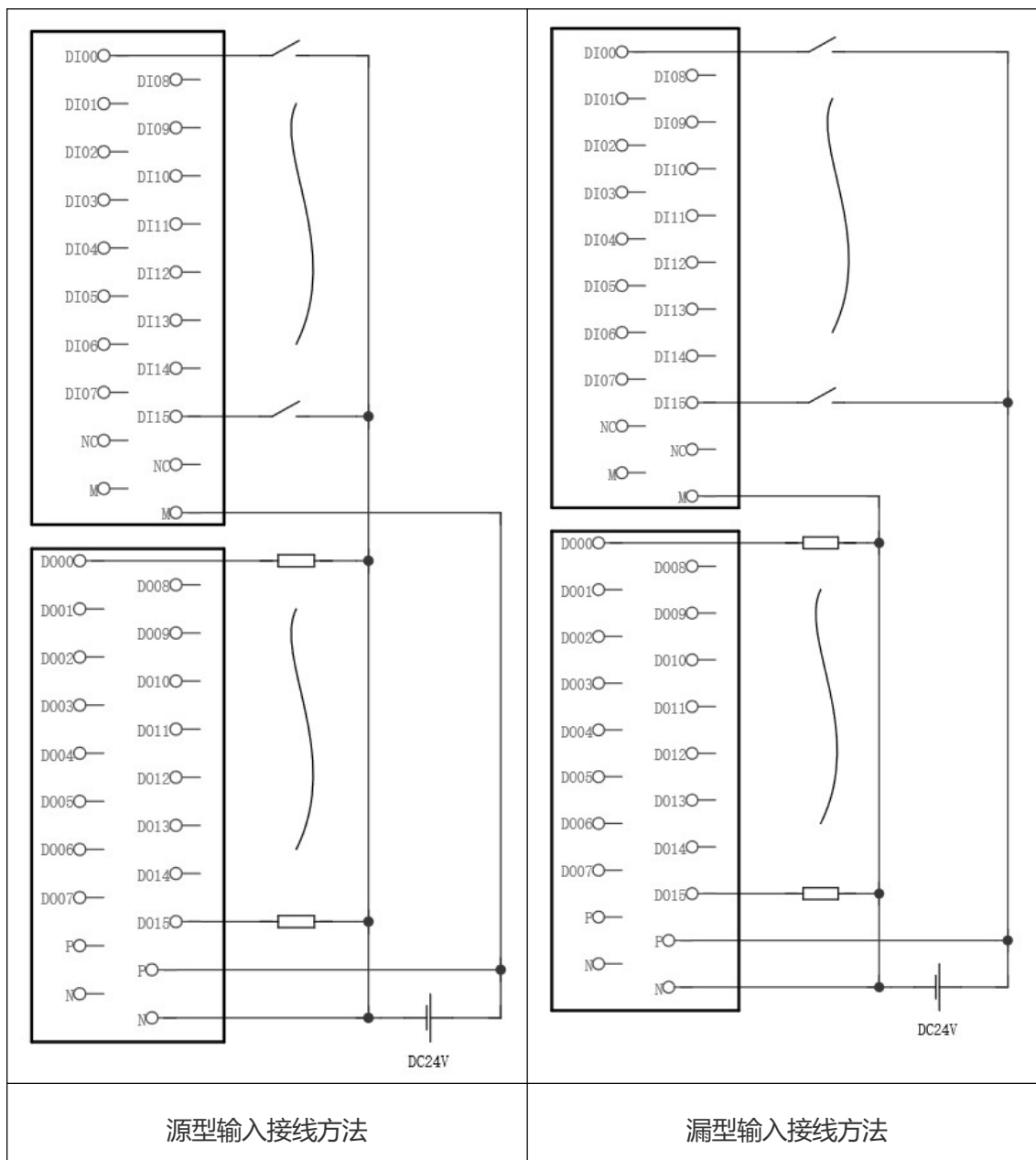
下图为 NPN 型数字量输入输出模块，CB-D1616N 的接线示意图。
